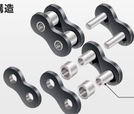
ラムダチェーン 基本構造
